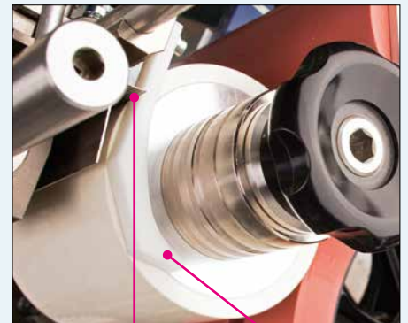
Img.: Cuchilla para impresión rotativa y rascador POM junto con un cliché cilíndrico, garantizan fiabilidad y un proceso de funcionamiento estable
