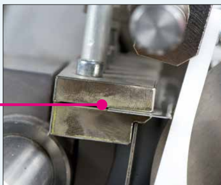
Img.: Vista detallada de la cuchilla de impresión rotativa integrada en el soporte para la cuchilla
